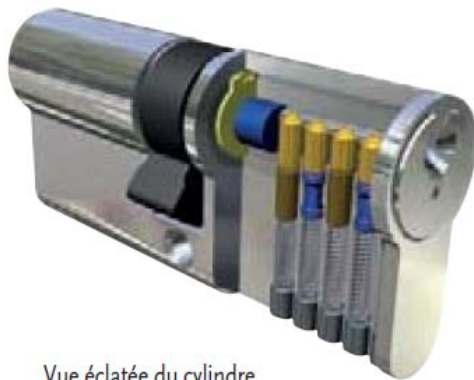
Vue éclatée du cylindre
