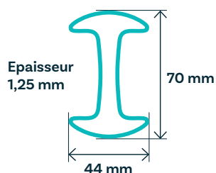
Section du poteau
