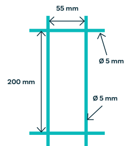
Dimensions des panneaux compatibles
